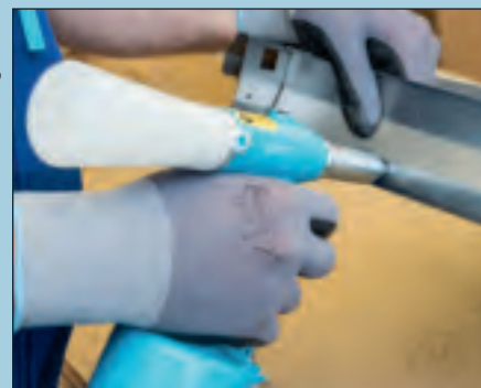
Mit Niet- und Mundstückschablone auf der Unterseite der Nietpistole
